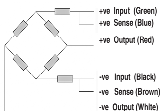
配线图
