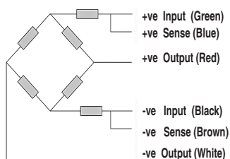
配线图
